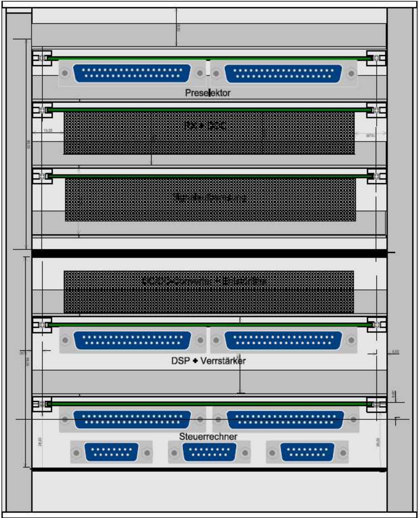
Bild 7 So wird der HSDR-4512 aufgebaut sein, wenn er fertig ist.
