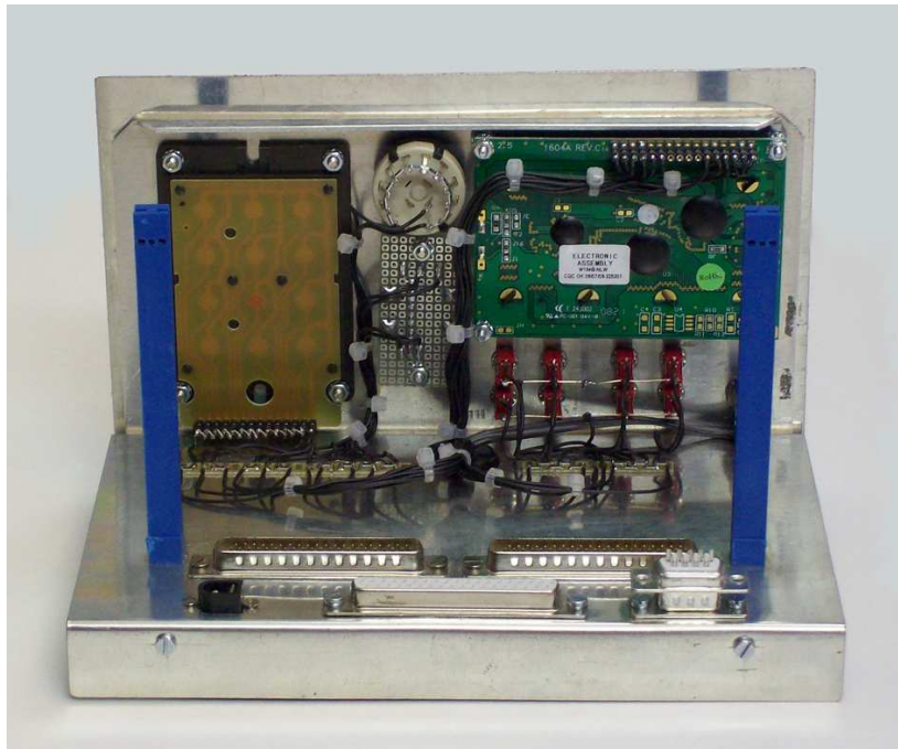
Bild 1 Hier sieht man die Verdrahtung der Frontplatte
