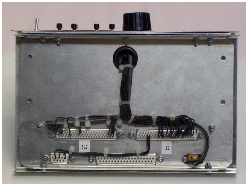
Bild 2 Die Verdrahtung der Unterseite
