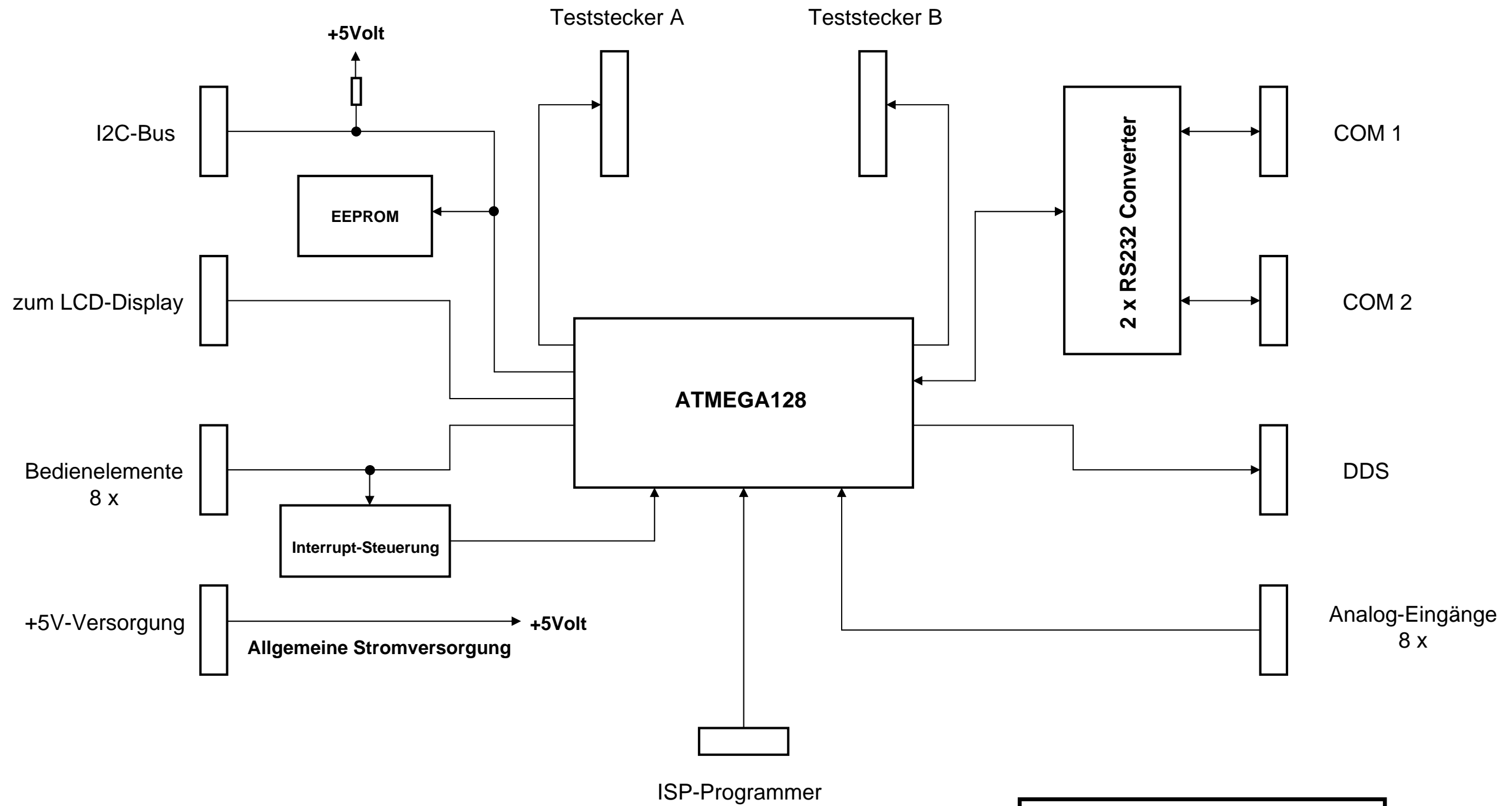
Blockschaltbild Steuerrechner HSDR-4512 24.12.2007 Werner, DL7MWN
