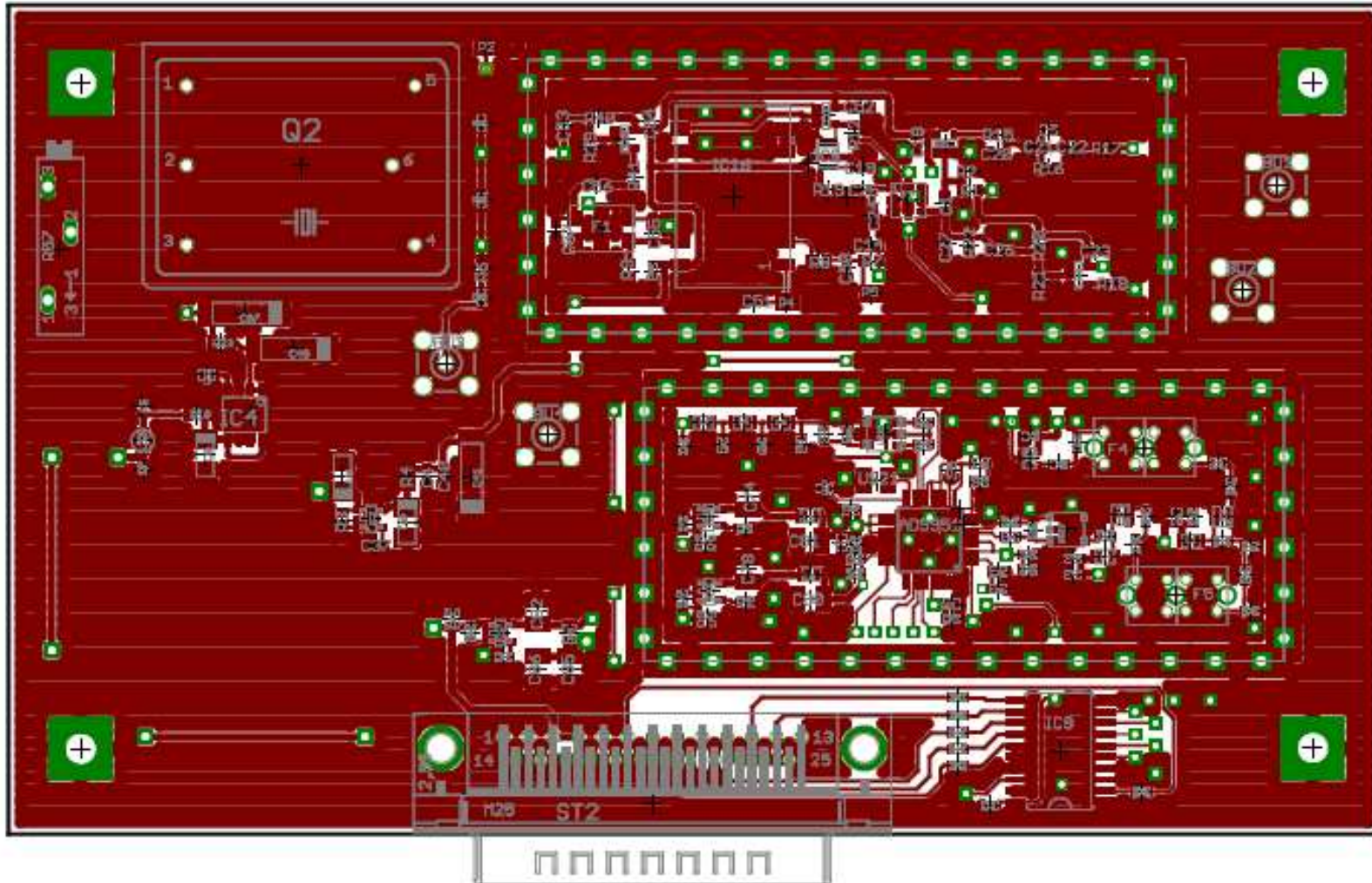
14.06.2009 BAVARIX Synthesizer Clock Bestückungsseite mit Massefläche
