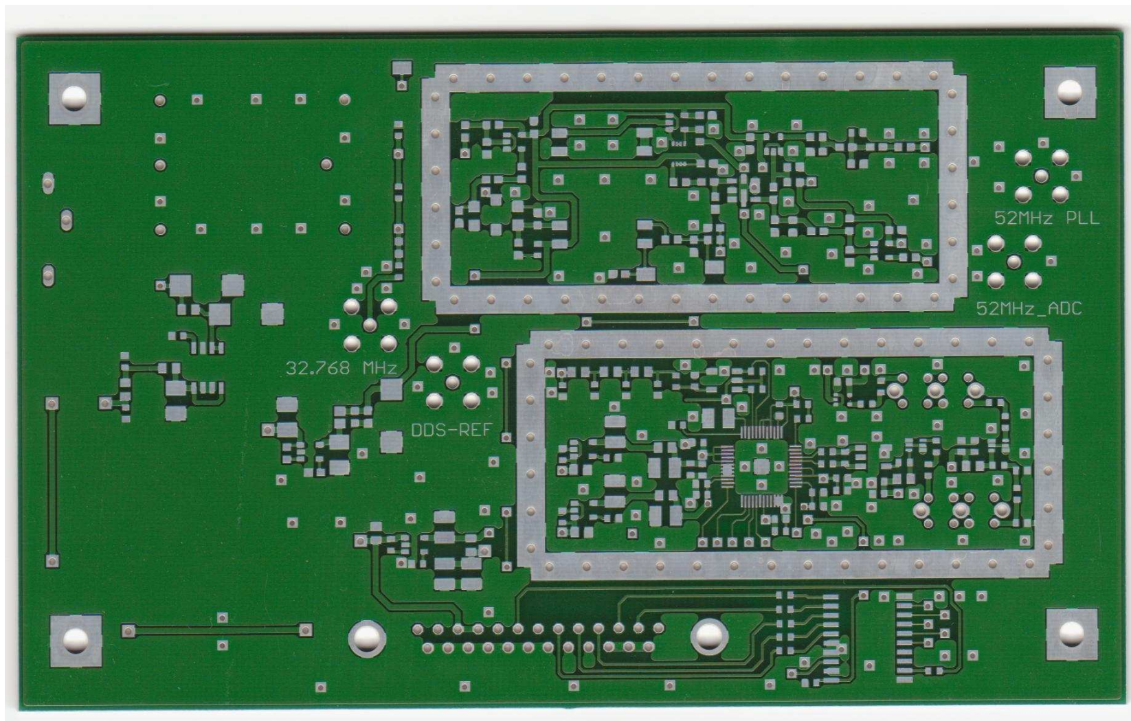
BAVARIX Synthesizer CLOCK - Oberseite
